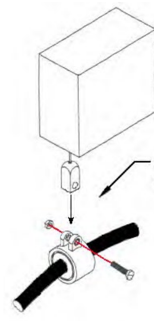
Illustration 2-3 Installation du serre-câble au rétracteur de câble
