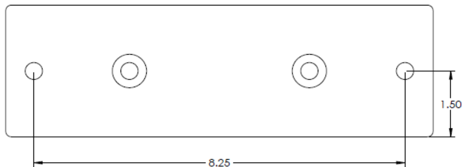
Illustration 2-1 Emplacements des trous de vis du support de fixation (2)
