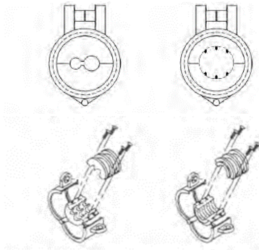
Illustration 2-2 Installation du serre-câble
